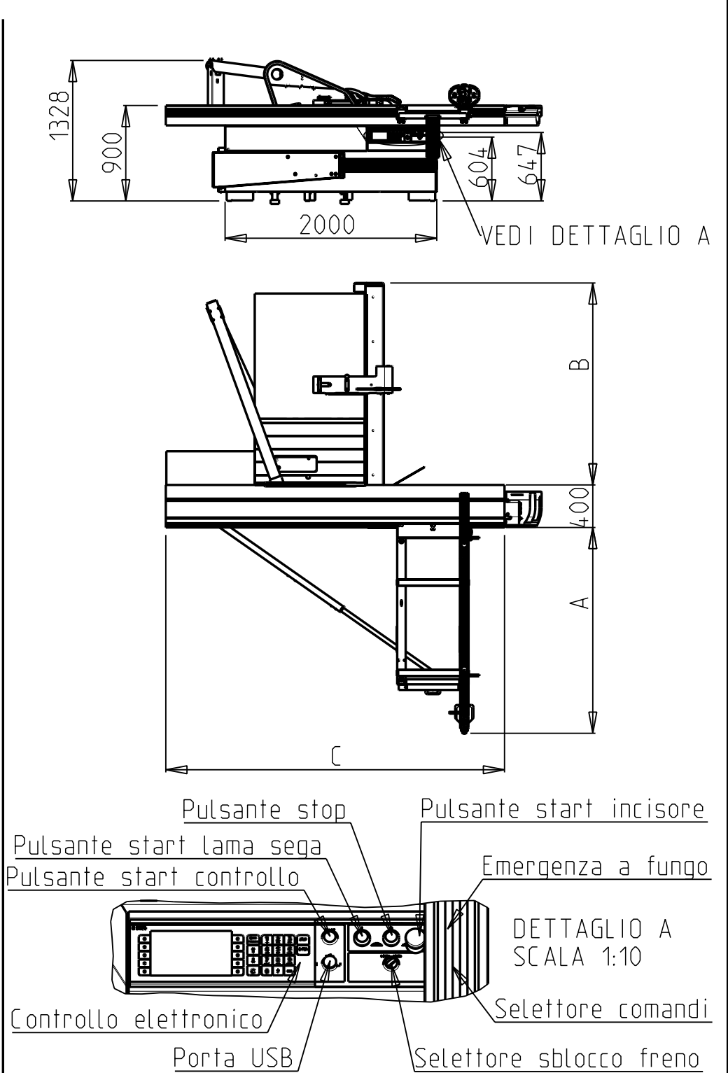
VERSIONE SENZA QUADRO PENSILE
