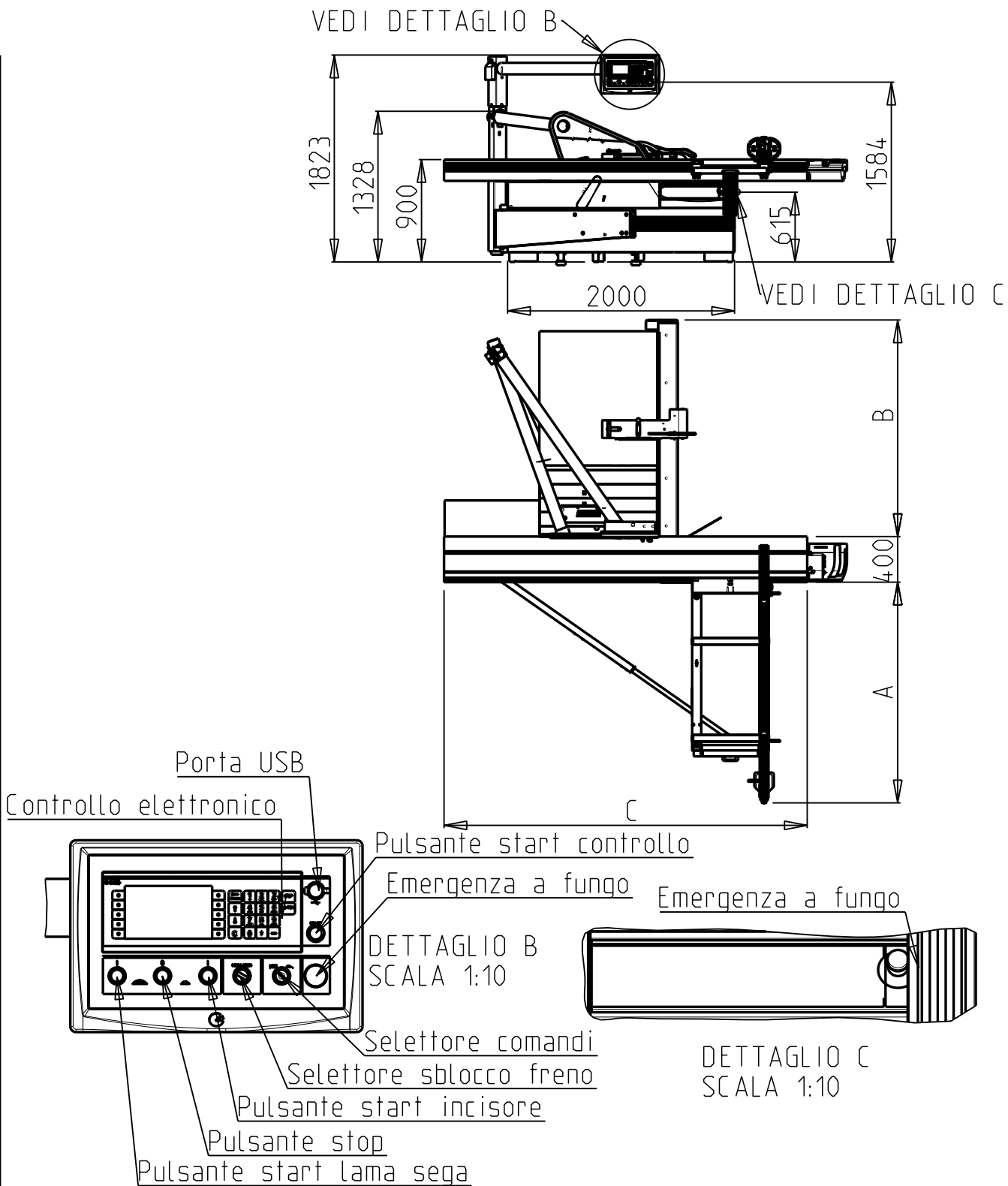
VERSIONE CON QUADRO PENSILE
